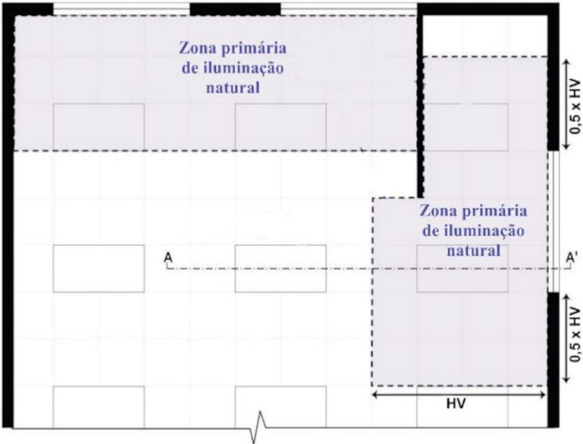
Figura 7.1 - Esquema em planta da definição zonas primárias de iluminação natural para as aberturas laterais
