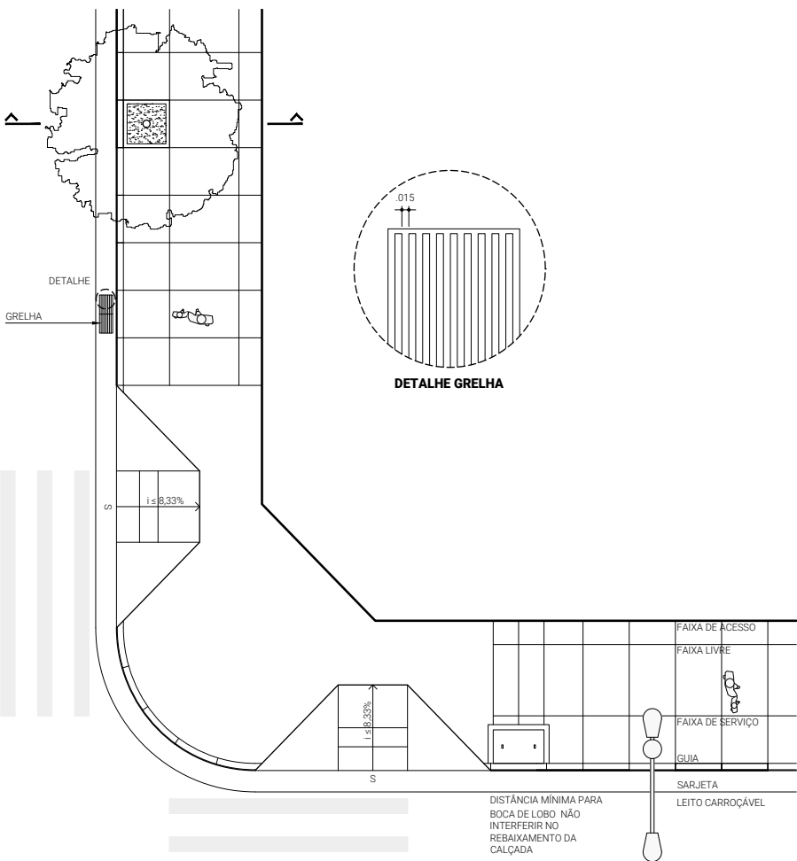
PLANTA
