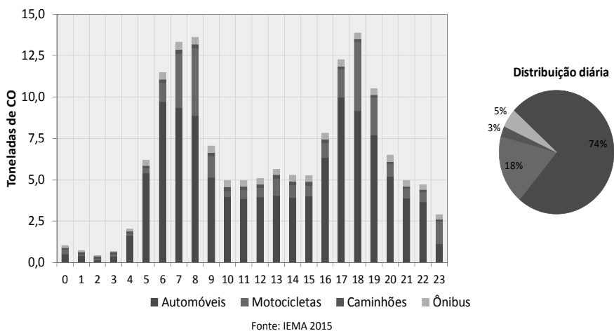
Gráfico 12 – Perfil horário médio das emissões de CO por categoria de veículo em dias úteis
