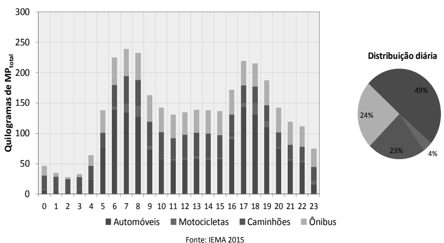
Gráfico 17 – Perfil horário médio das emissões de MPtotal por categoria veicular em dias úteis
