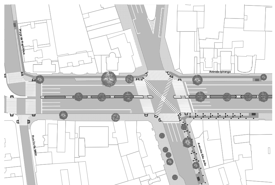
Figura 20 – Exemplo de projeto básico de uma conexão, em desenvolvimento na SPTrans
