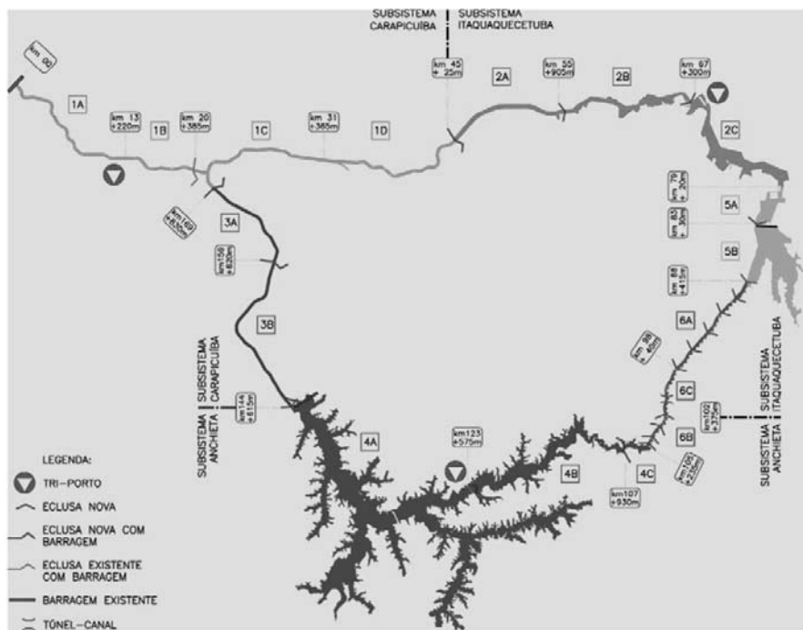
Figura 32 – Diagrama dos trechos do Hidroanel Metropolitano
